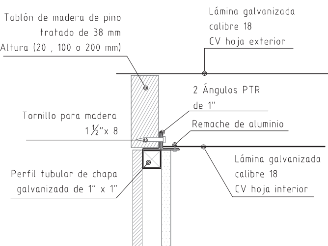
Detalle 11
