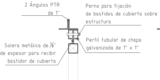
Detalle 08
