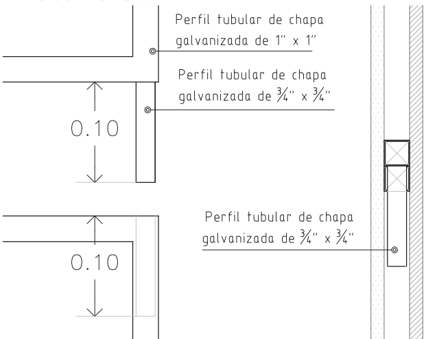
Detalle 06
