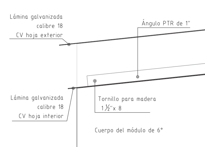
Detalle 10
