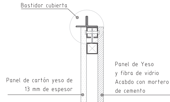
Detalle 10
