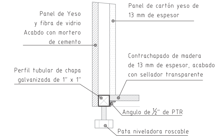
Detalle 03
